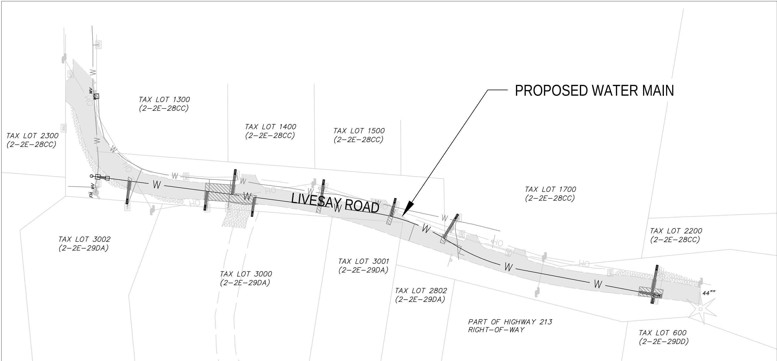
SITE MAP SCALE: 1" = 50' (22"X34")
