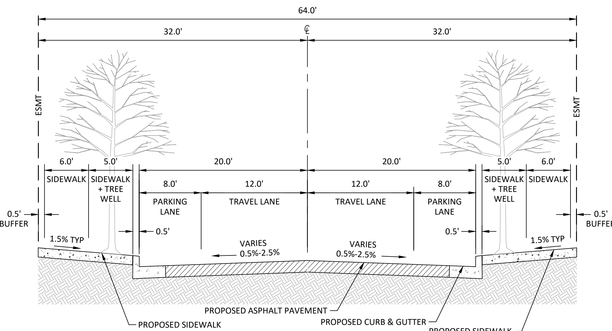
INTERNAL ROADS N.T.S.
